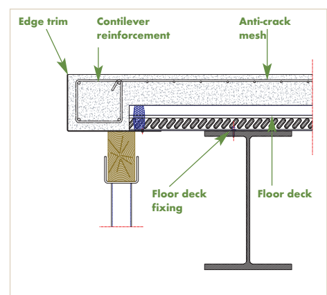
Prop under edge trim
