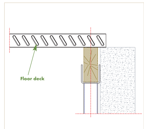
Edge prop
